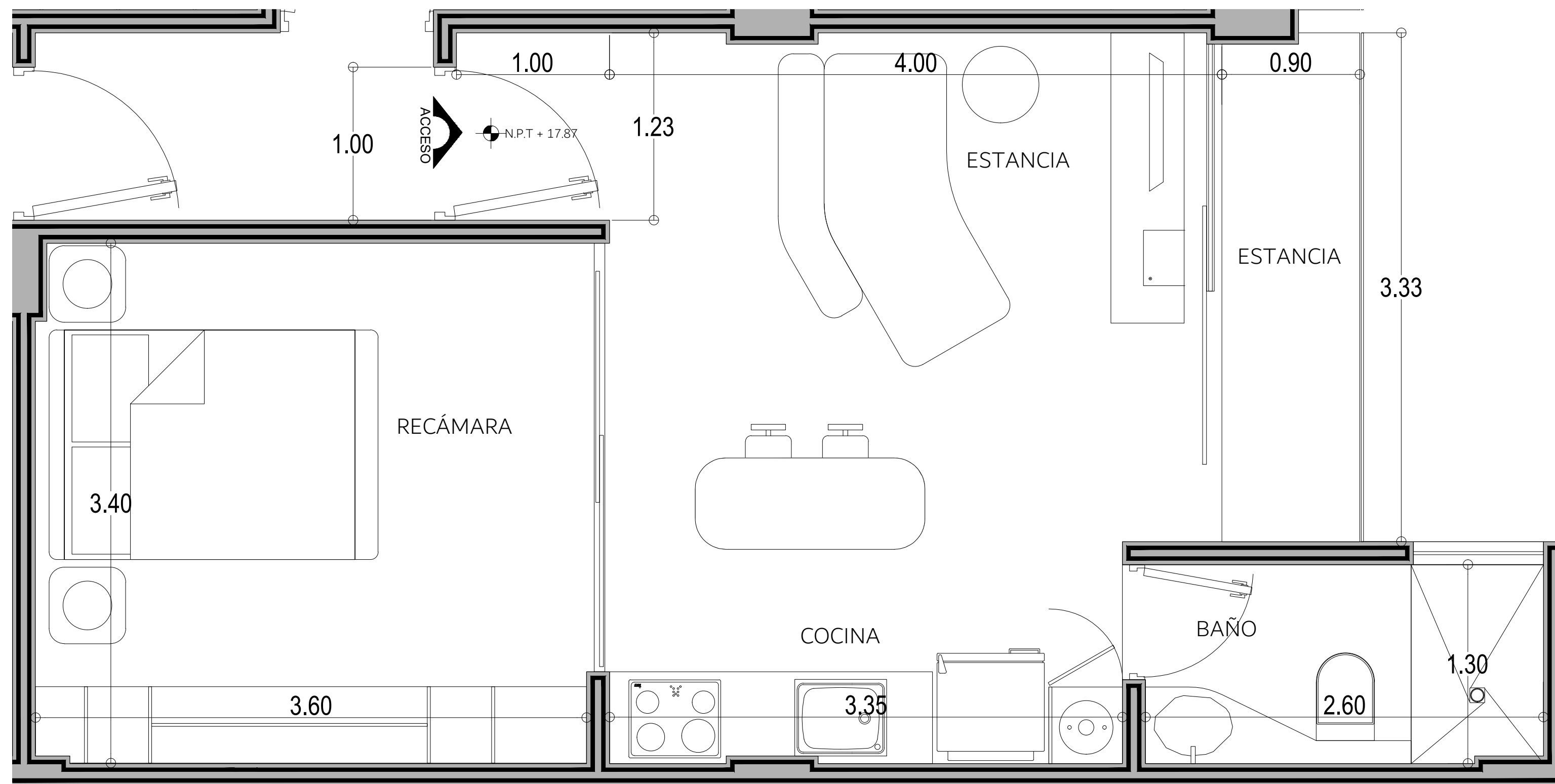
PLANTA ARQUITECTÓNICA DEPARTAMENTO C603 ESCALA 1:10
