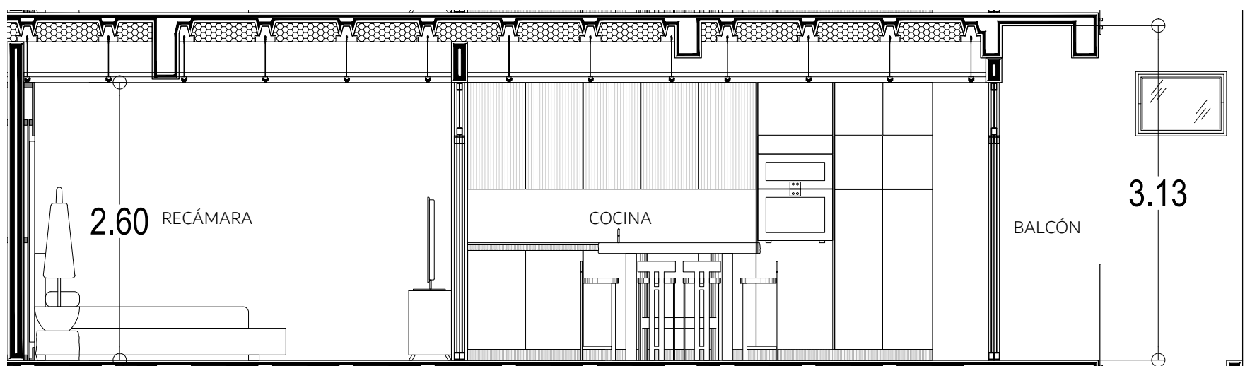
CORTE LONGITUDINAL A-A DEPARTAMENTO B402 ESCALA 1:20
