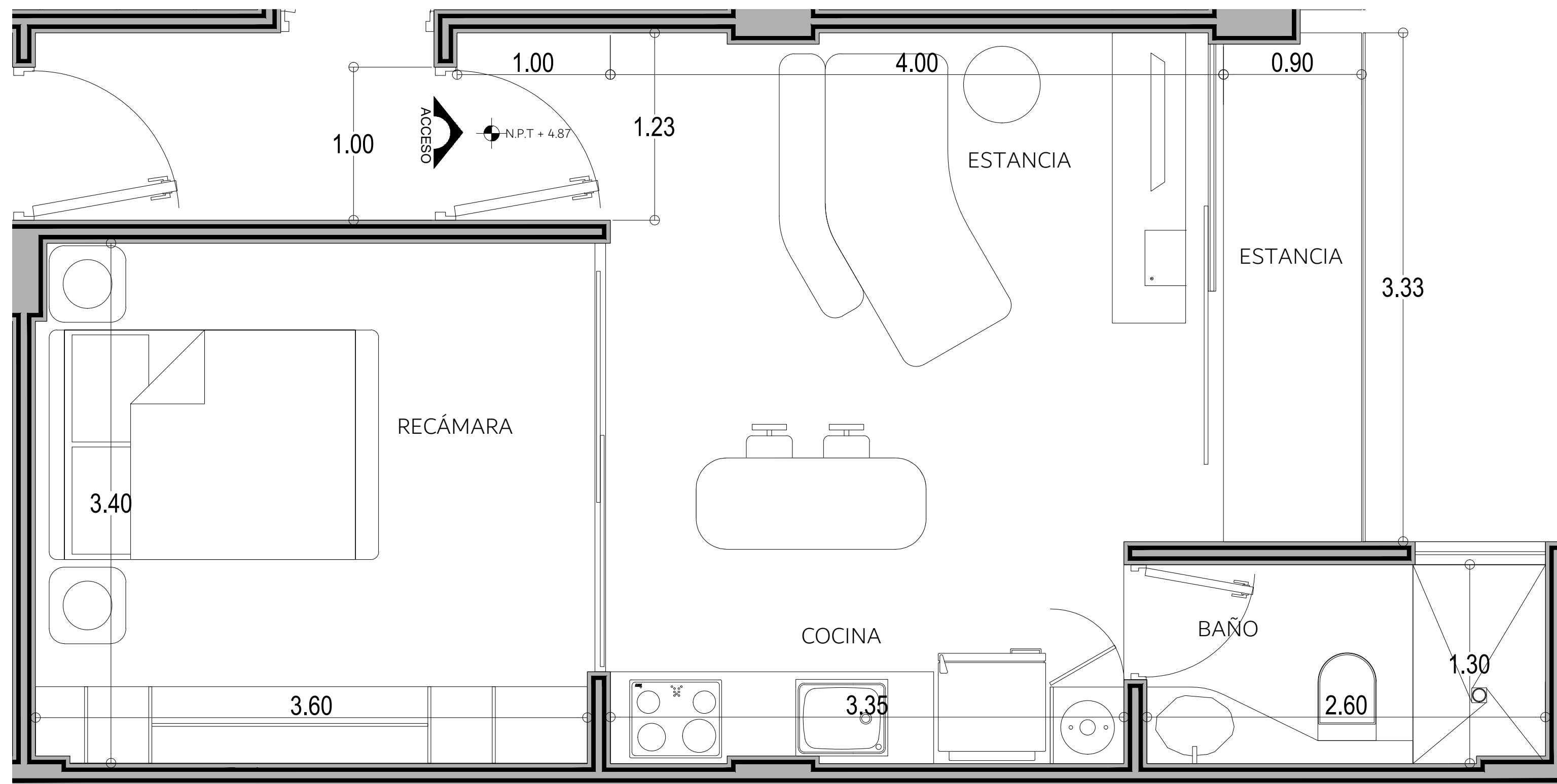
PLANTA ARQUITECTÓNICA DEPARTAMENTO C103 ESCALA 1:10
