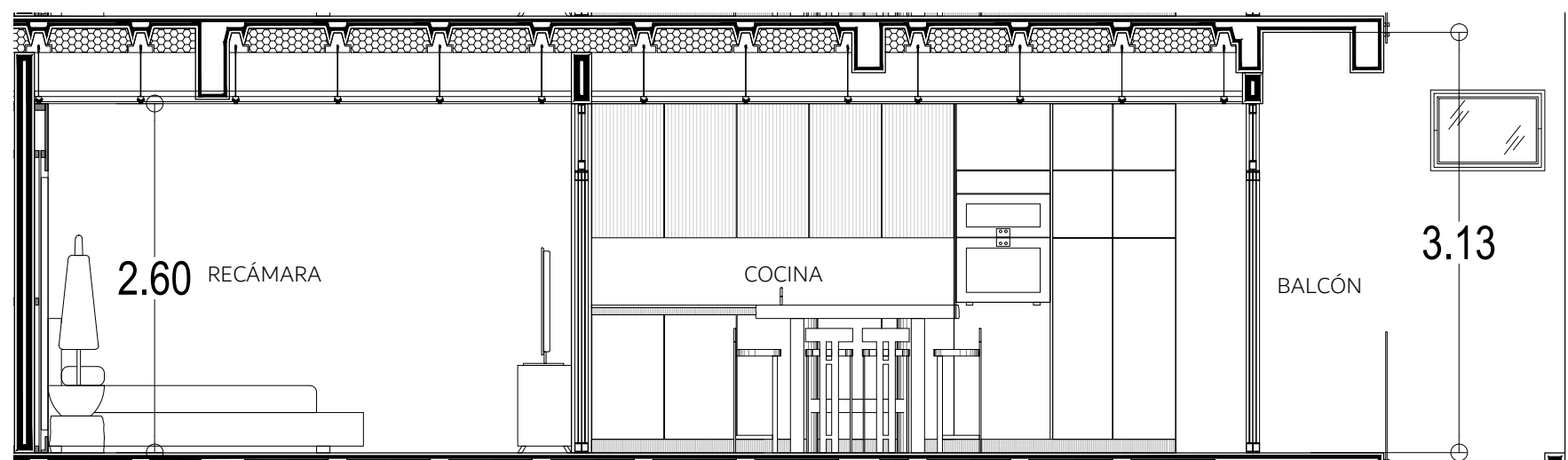
CORTE LONGITUDINAL A-A DEPARTAMENTO B102 ESCALA 1:20
