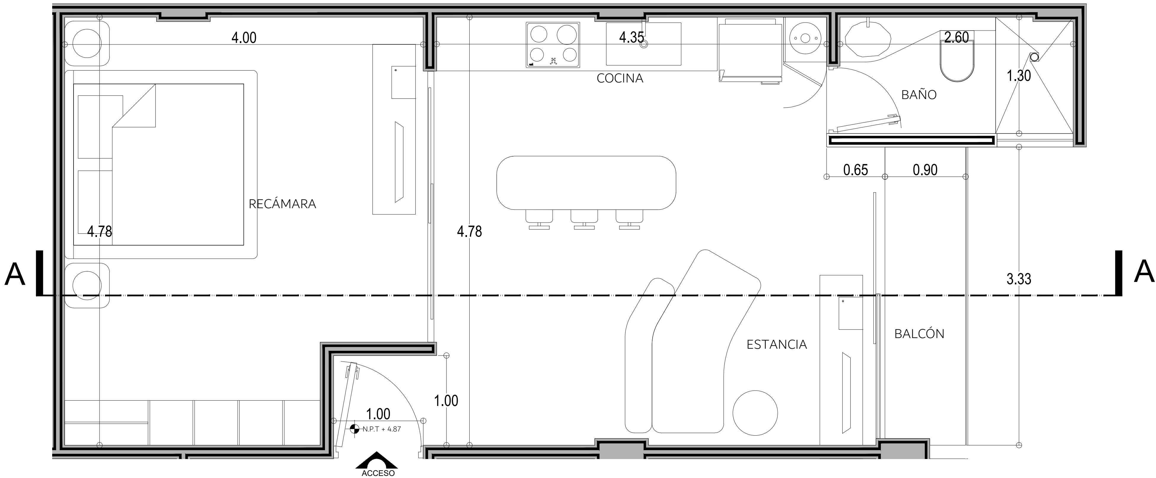
PLANTA ARQUITECTÓNICA DEPARTAMENTO B102 ESCALA 1:10
