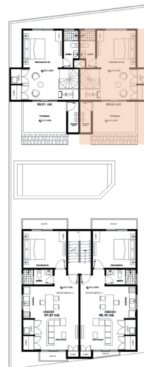
PLANTA NIVEL DOS
