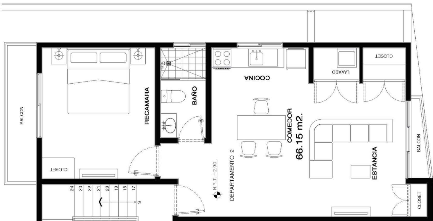
NIVEL UNO DEPARTAMENTO 2
